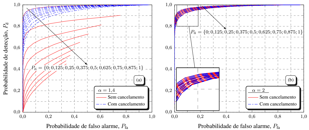
Figura 1.2: ROCs do detector GRCR sob ruído impulsivo S\alpha S com e sem cancelamento, para \alpha = 1,4 (a) e \alpha = 2 (b), para \gamma = 1 e diversos valores de P_{ri} .
